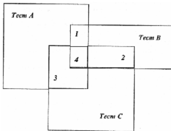
Рис. 5. Модель факторного анализа
